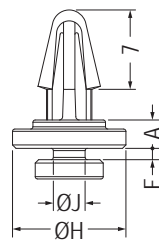
【ACB-2.3】
