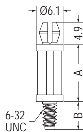
【 MSPS-13 】
