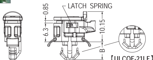
【ULCOF-21LF】
