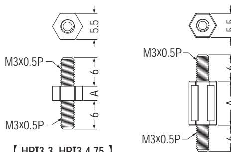
【 HPI3-3, HPI3-4.75 】
