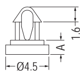
【 MAM-1.5L 】
