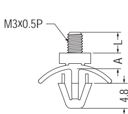
【 LCDS3-3, LCDS3-4 】
