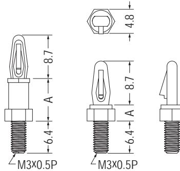
【 SCB3-12.7 】
