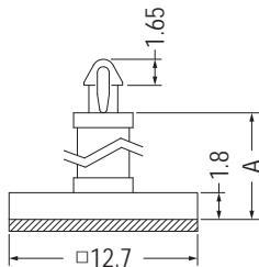
3M DOUBLE ADHESIVE TAPE A 尺寸不含背膠高度
