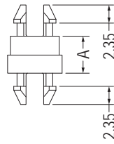
【 MSPK4.8-4.8 】
