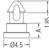
【 MAM-2.6 】
