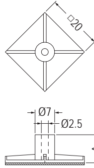
3M DOUBLE ADHESIVE TAPE A 尺寸不含背膠高度
