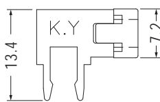
【 PCB-4F 】
