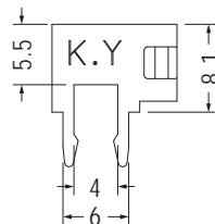
【 PCB-4 】
