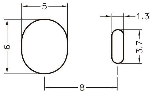
HOLE IN P.C.B
